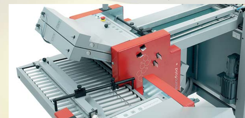
La station pli croisé. Tous les modèles Eurofold peuvent être équipés avec une station pli croisé à tout moment.
