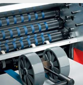
Les cylindres mixtes avec entraînement par pignons hélicoïdaux.
