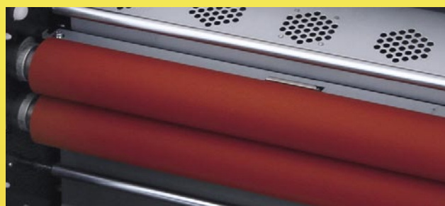
Système par rouleaux chauffants avec résistances haute performance
