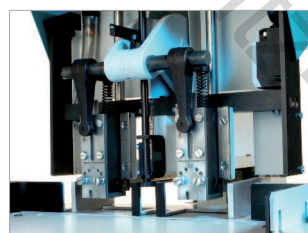
Écartement réglable des têtes d'agrafage de 80 à 155 mm.
